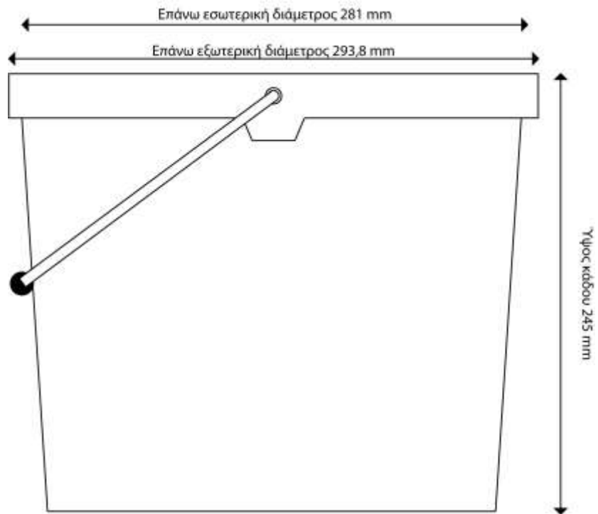
Σχέδιο 1. Διαστάσεις πλαστικού κάδου
