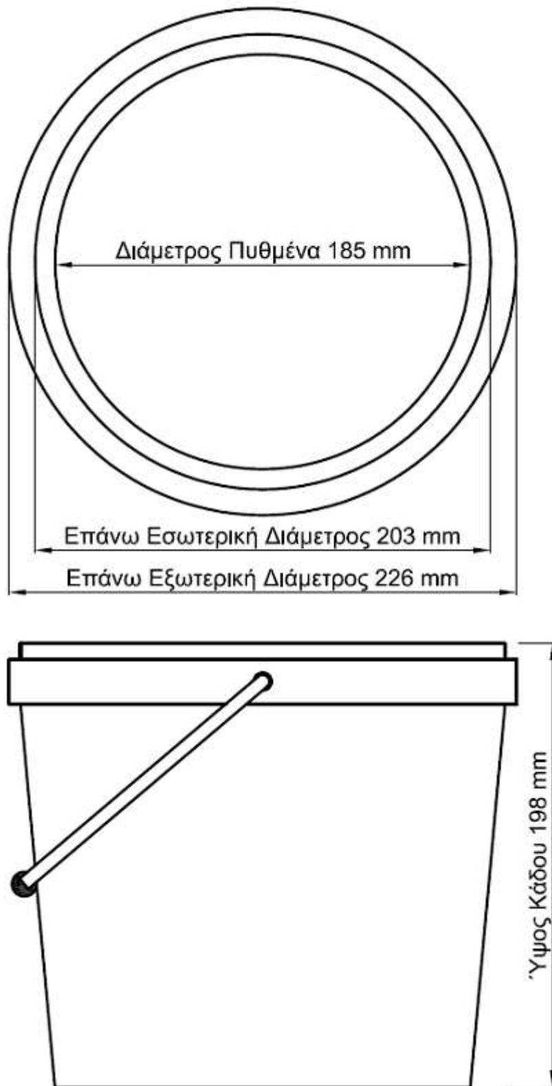
Σχέδιο 1. Διαστάσεις πλαστικού κάδου
